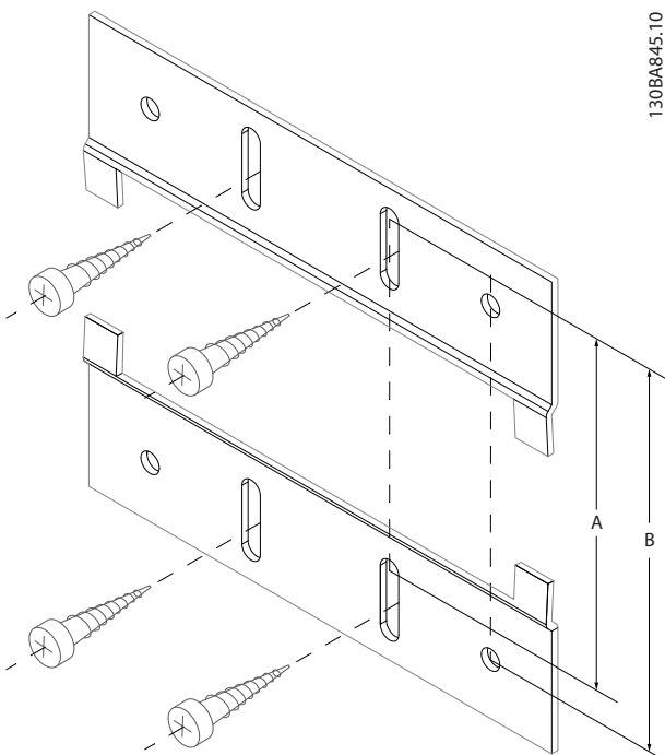
图 11.31 上托架
