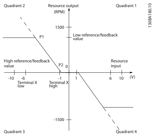
图 3.20 反向死区
