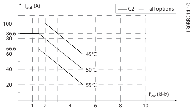
图 6.33 输出电流在不同开关频率和环境温度下的降容 - 机箱类型 C2, SFAVM。注意：图中的电流为绝对值，且对高过载和正常过载都有效。
