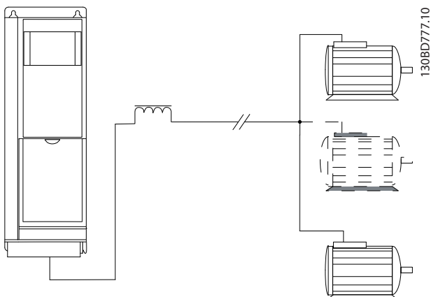
图 9.53 带负载的并行电缆
