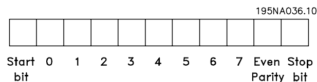
图 12.5 字符内容
