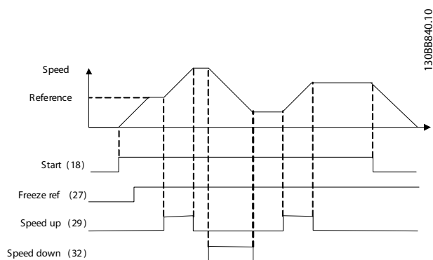
图 10.3 加速/减速
