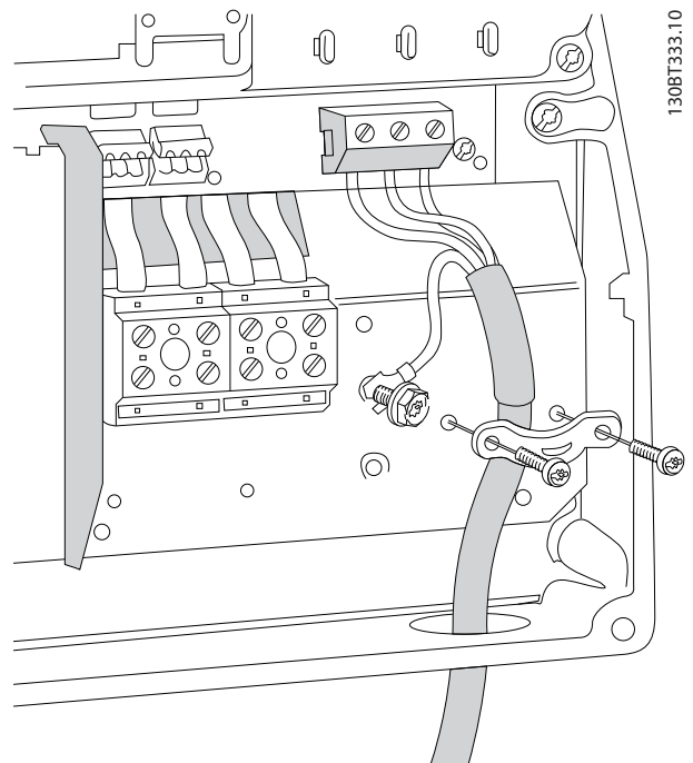
图 9.32 机箱 B1 和 B2 的电动机接线
