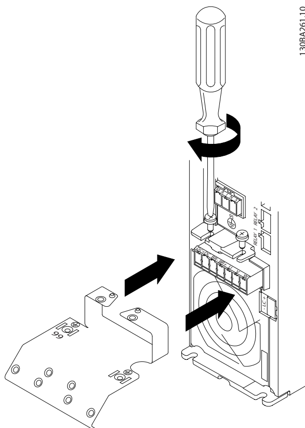
图 9.17 支撑板
