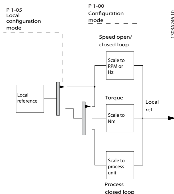
图 3.12 配置模式
