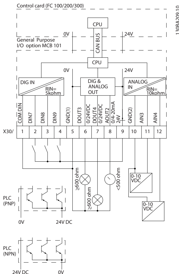
图 11.2 原理图
