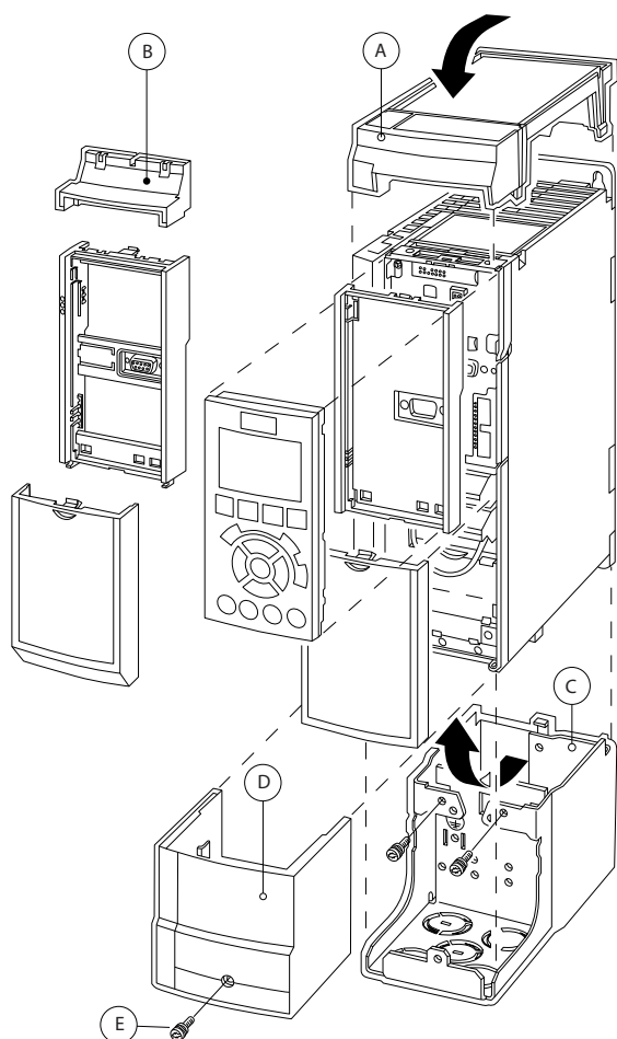
图 11.23 机箱类型 A2
