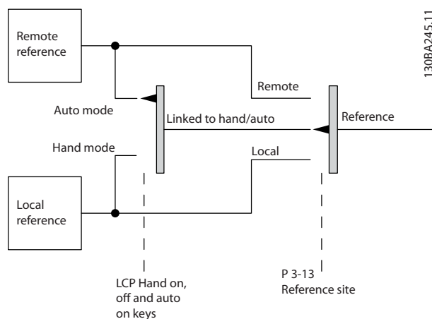
图 3.11 有效参考值
