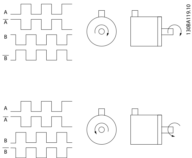
图 11.5 旋转方向
