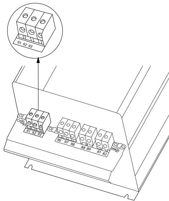
图 9.27 主电源连接机箱 C3 (IP20)
