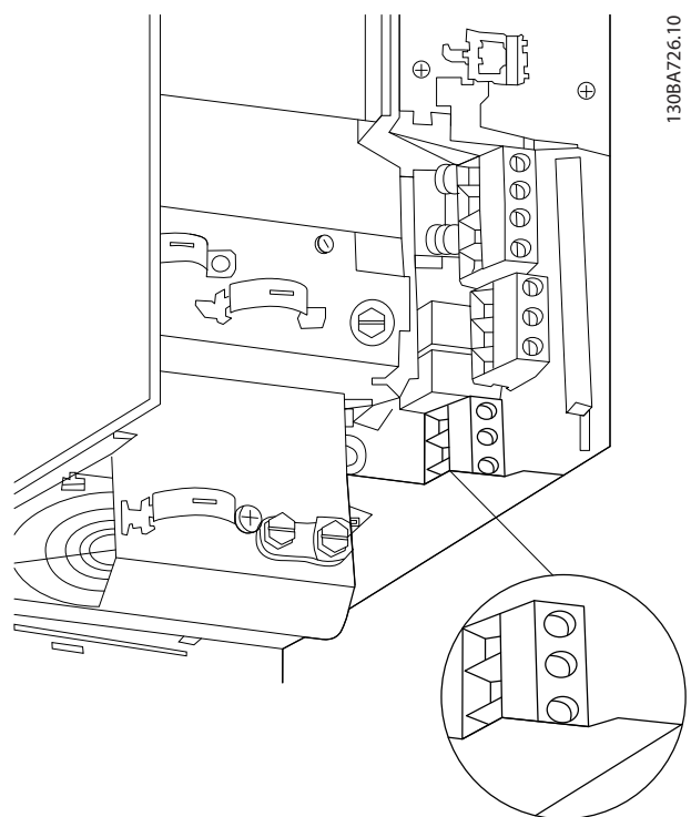
图 9.33 机箱 B3 的电动机接线
