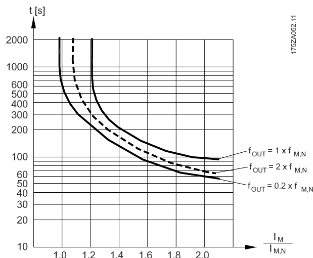
图 4.1 ETR 特性
