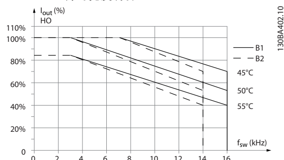
图 6.6 I_{out} 在不同 T_{AMB, MAX} 下的降容, 机箱类型 B1 和 B2, 在高过载模式 (160% 过转矩) 下使用 60° AVM
