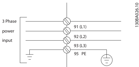
图 9.16 主电源接线
