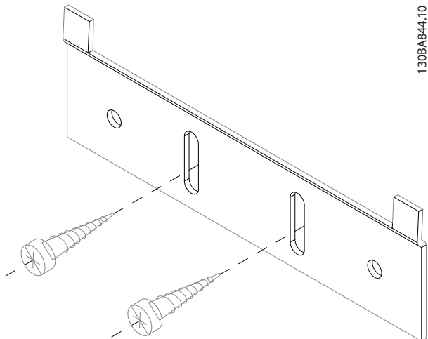
图 11.30 下托架
