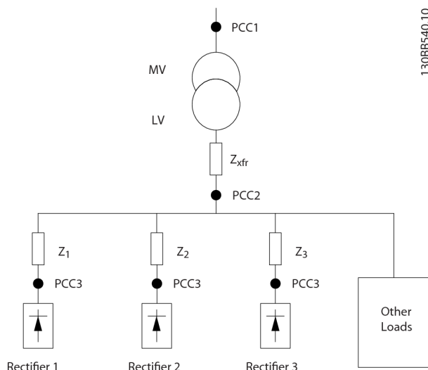
图 5.5 小配电系统
