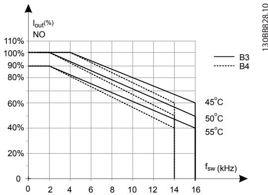
图 6.9 I_{out} 在不同 T_{AMB, MAX} 下的降容, 机箱类型 B3 和 B4, 在正常过载模式 (110% 过转矩) 下使用 60^\circ AVM
