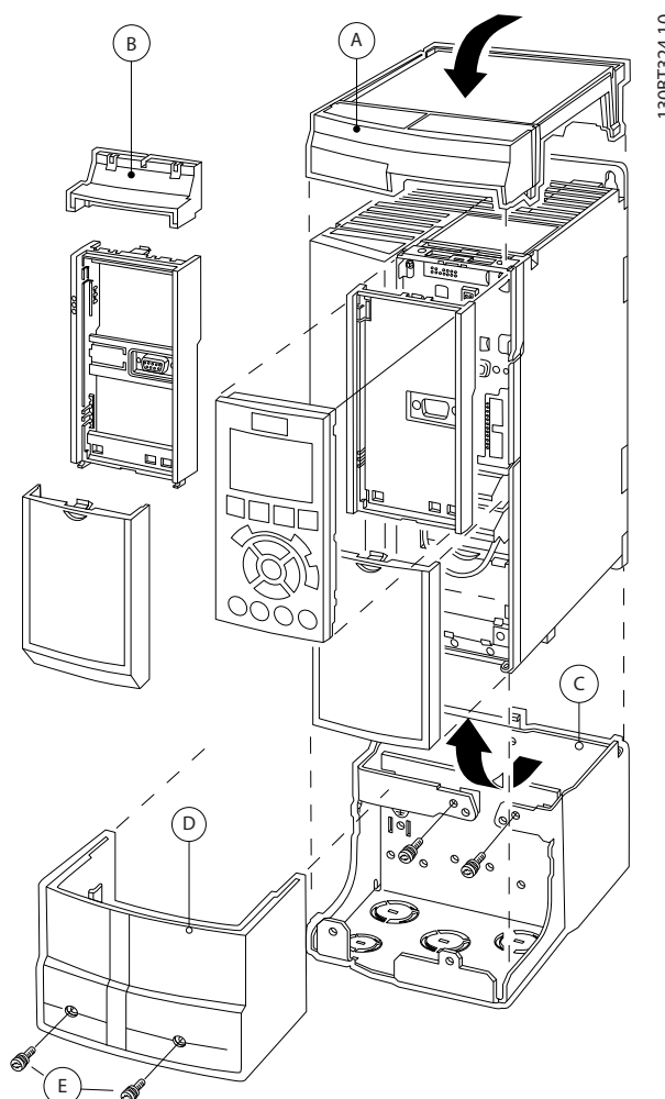
图 11.24 机箱类型 A3
