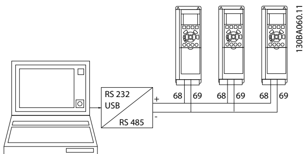
图 12.2 并行连接
