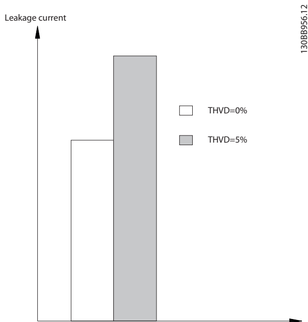
图 9.38 线路失真会影响漏电电流
