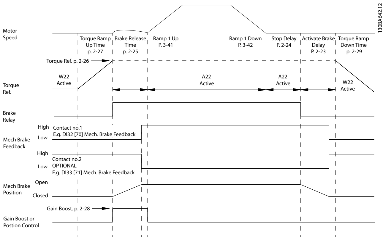
图 4.3 起重机械制动控制的抱闸释放过程 此制动控制仅在带电动机反馈的磁通矢量中可用，对于异步和非突出 PM 电动机可用。
