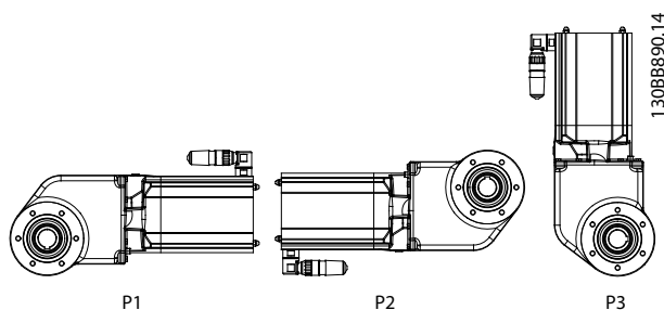
图 4.8 OneGearDrive
