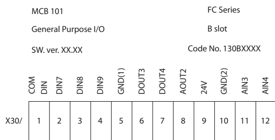
图 11.1 MCB 101 选件
