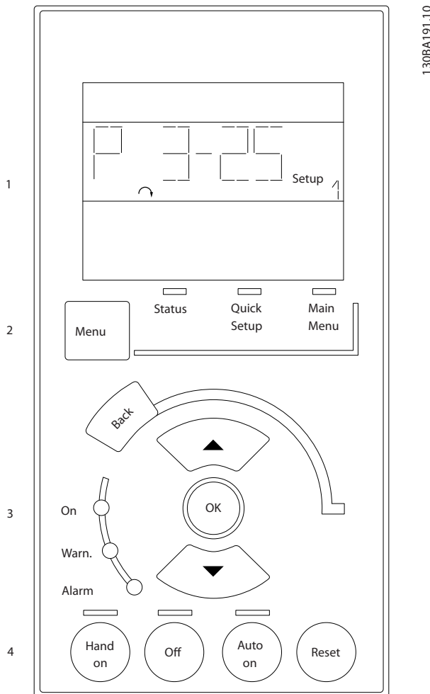
图 2.21 LCP 键
