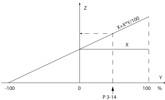
图 3.23 实际参考值
