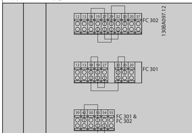
图 3.61 测试插头
