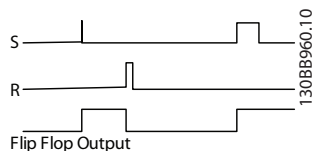
图 3.54 正反器输出
