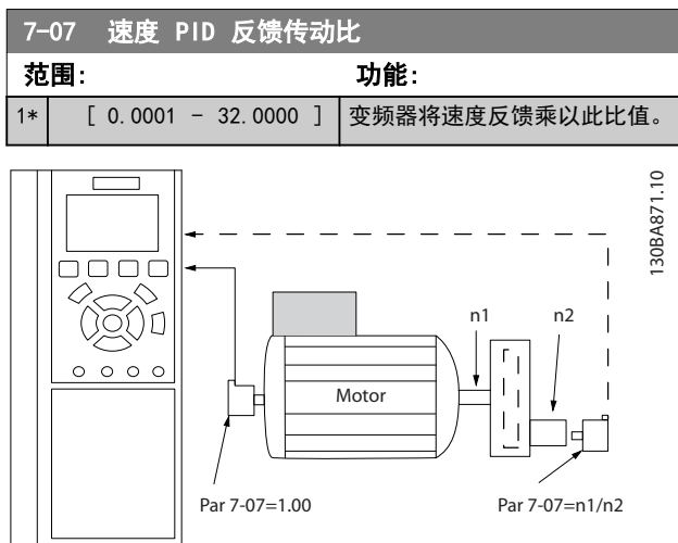
图 3.48 速度 PID 反馈传动比
