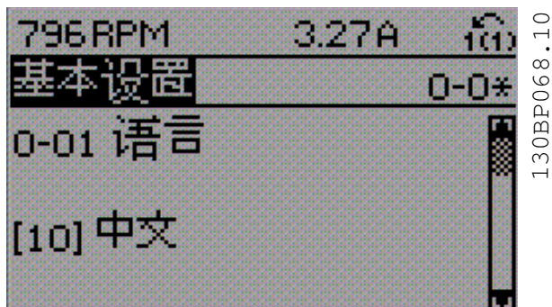
图 2.16 更改文本值
