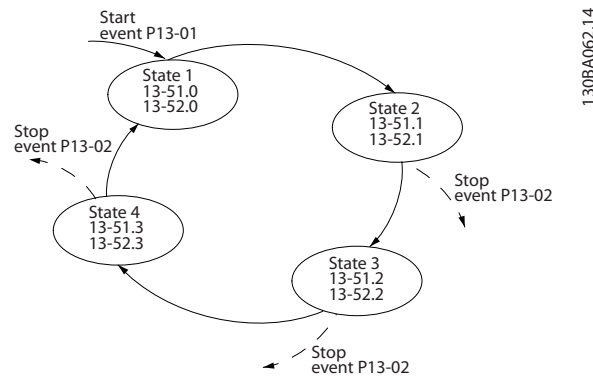
图 3.51 事件和操作
