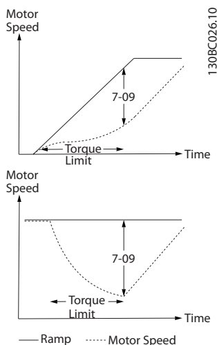
图 3.49 加减速和实际速度之间的速度误差
