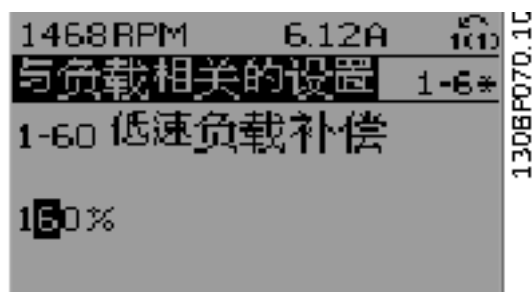
图 2.18 保存数据值
