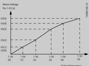
图 4.3 U/f 特性示例
