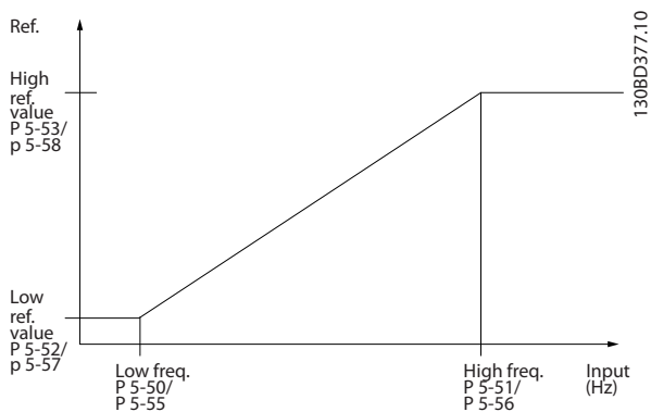
图 4.14 脉冲输入
