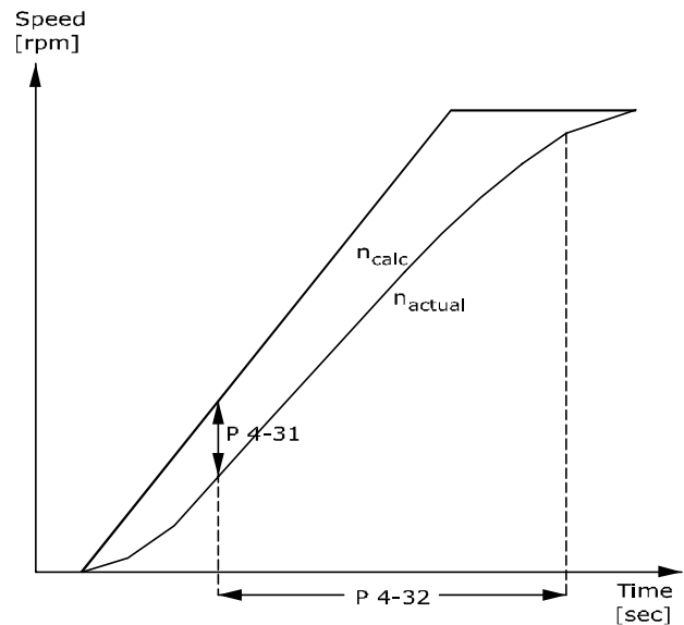
130BA221.10 图 4.10 电机反馈速度错误
