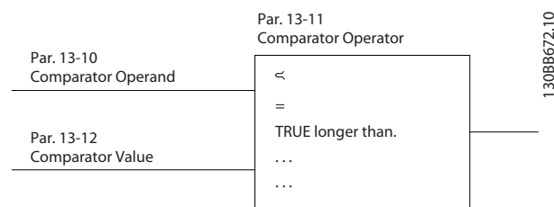
图 4.24 比较器
