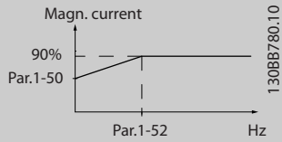
图 4.2 电动机磁化
