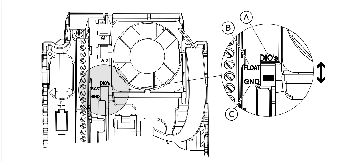
图 13: DIP 开关
