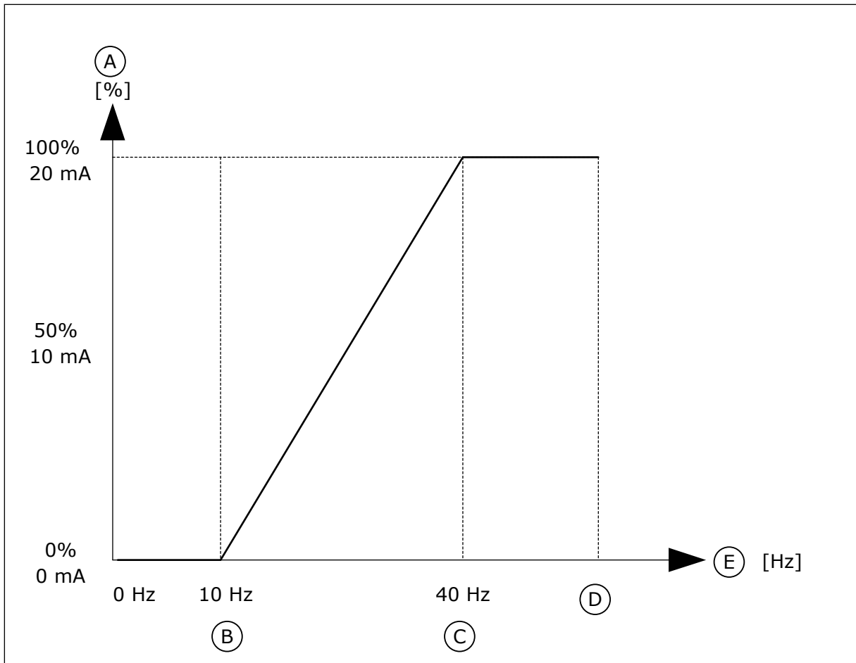
图 53: AO1 信号的缩放
