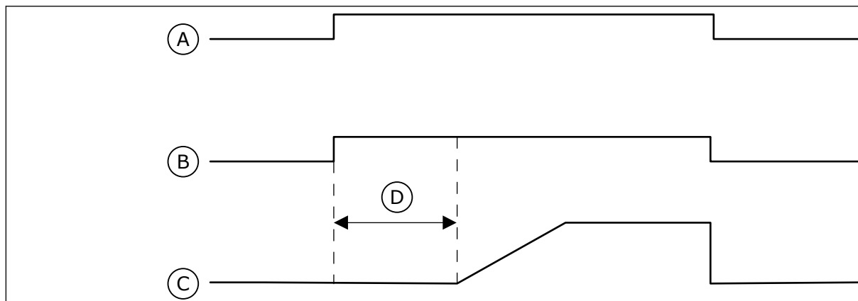
图 93: 注给泵功能
