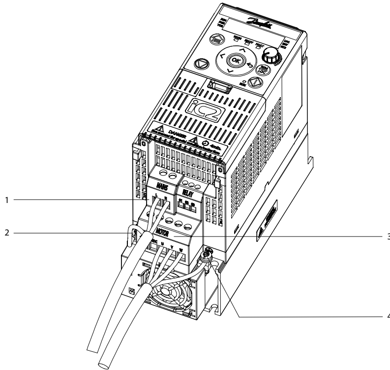
图解 37: 单相设备的主电源、电机和接地 j 接线 (以 MA02c 为例)
