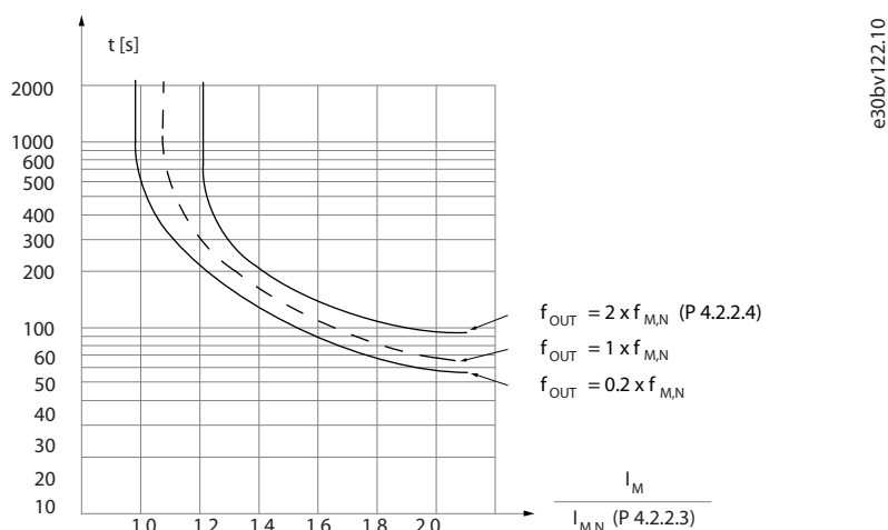
图解 36: ETR
