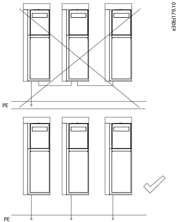
图解 32: 接地原理
