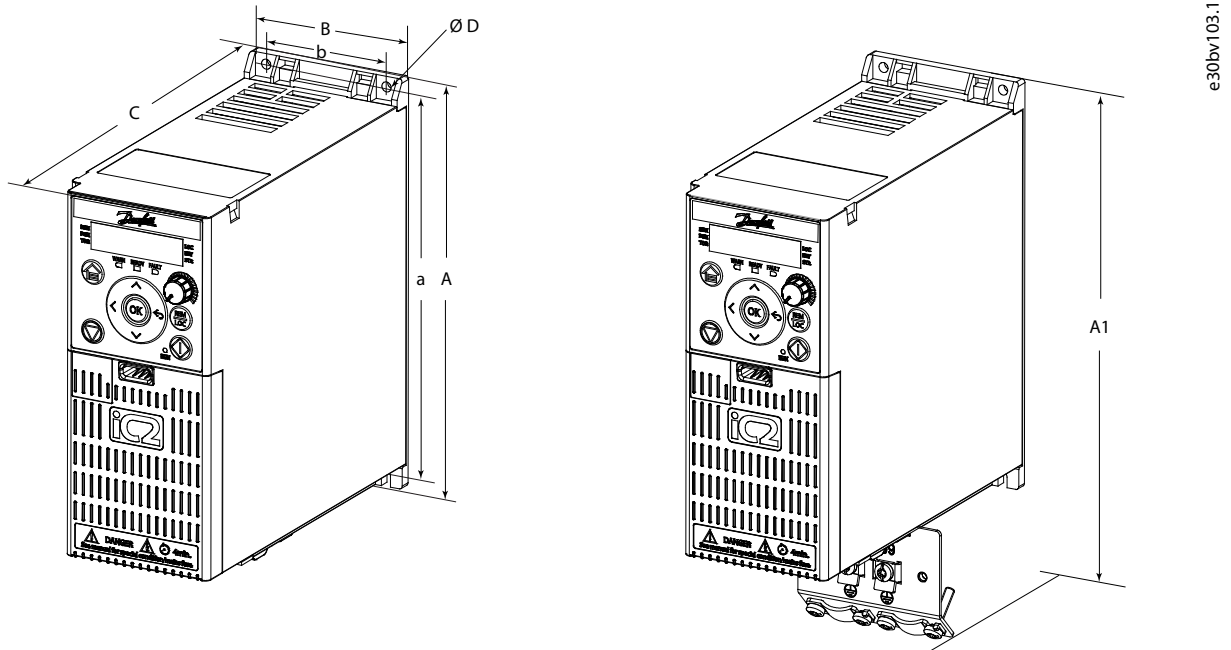
图解 18: IP20/开放型机箱规格和尺寸
