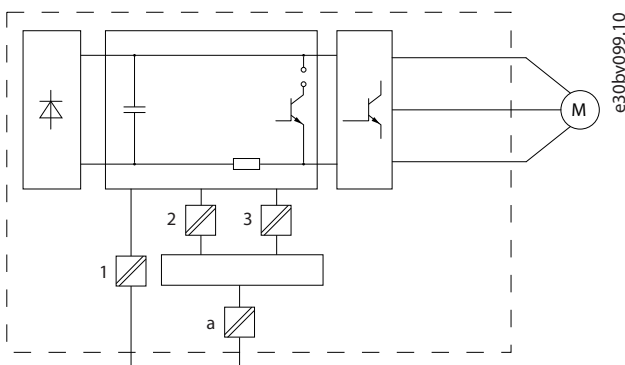
图解 33: 电隔离
