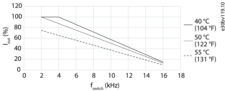
图解 15: 输出电流降额与开关频率的关系 (MA01a 3x380-480 V AC)
