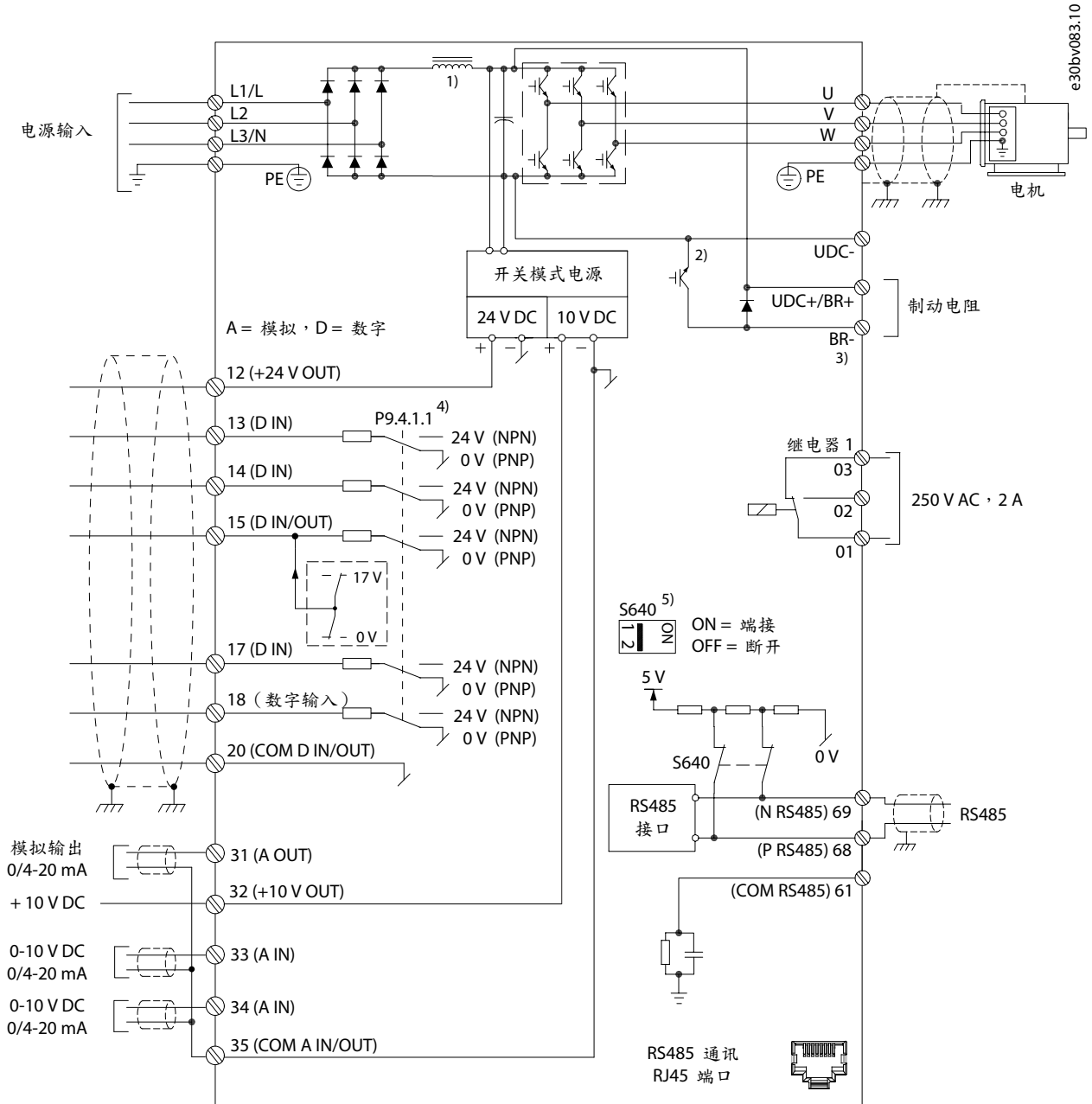
图解 28: 接线图
