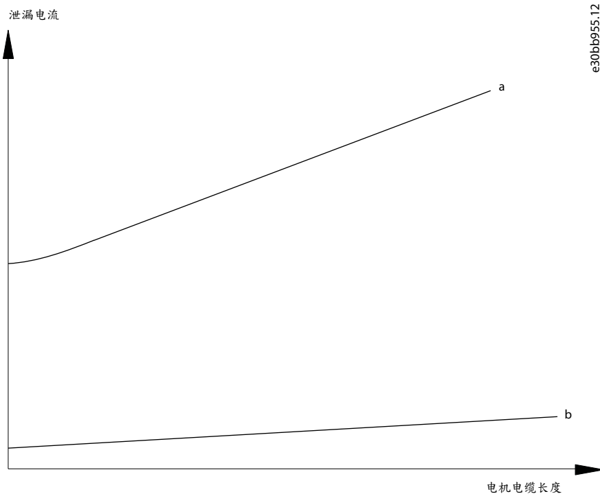
图解 34: 电缆长度和功率规格对漏电流的影响, P_a > P_b
