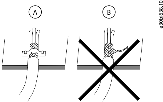
图解 31：安装电缆屏蔽层
