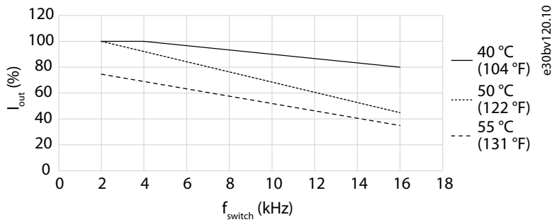
图解 16: 输出电流降额与开关频率的关系 (MA02a 1x200 - 240 V AC)
