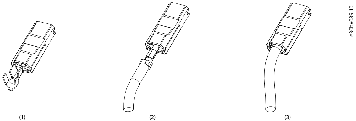
图解 43: 连接用于负载共享和制动的端子
