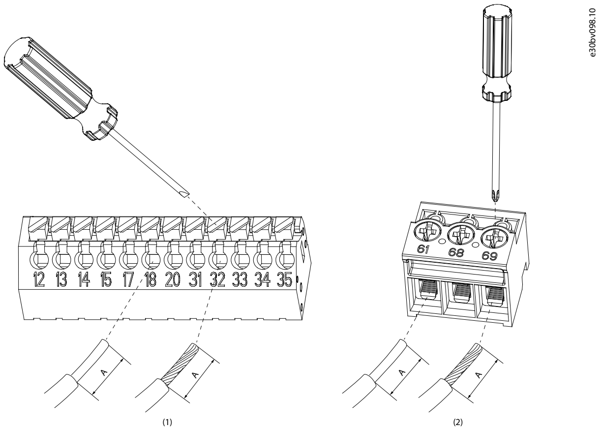
图解 41: 将线缆插入端子
