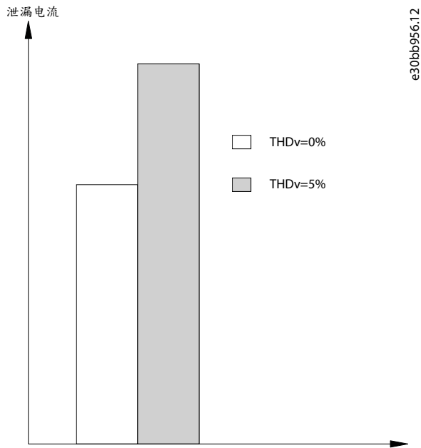
图解 35: 电网失真对泄漏电流的影响。
