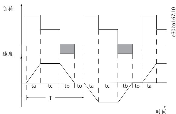
图解 12: 典型的制动周期
