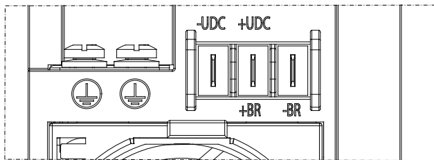
图解 45: MA02a 的制动功能 (3x380-480 V)
