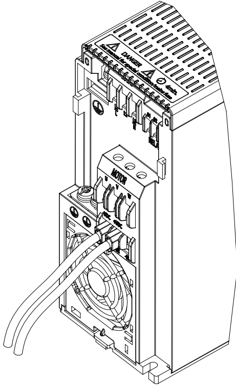
图解 44: 连接到负载共享和制动装置
