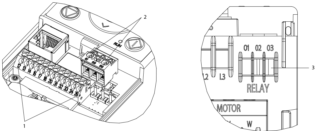
图解 40: 控制端子编号和位置
