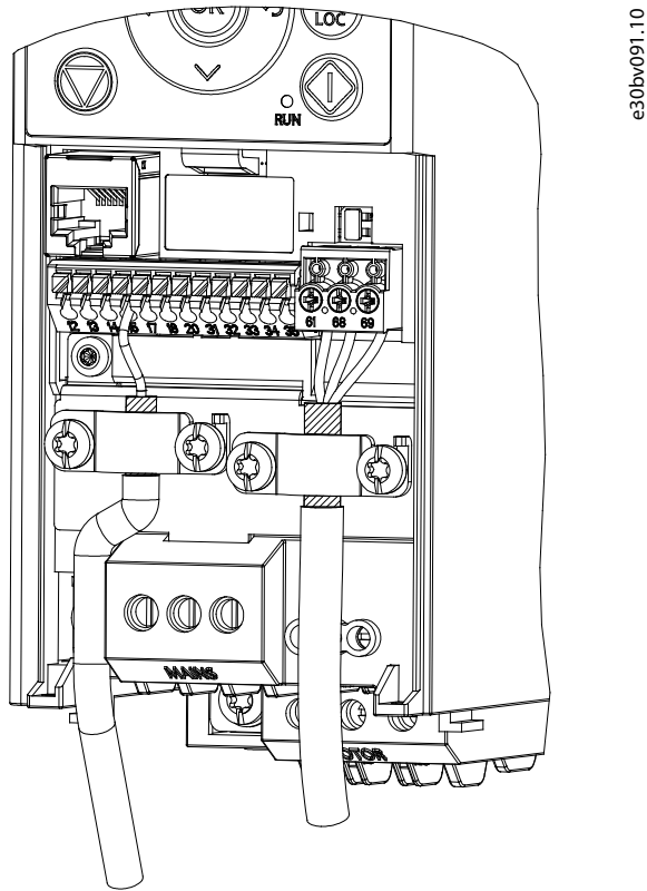
图解 42: 电缆屏蔽层的正确连接
