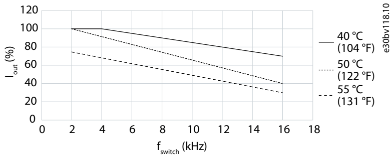
图解 14: 输出电流降额与开关频率的关系 (MA02c 1x200 - 240 V AC)
