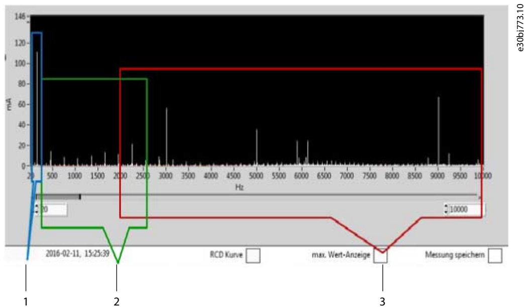
图解 29: FFT 测量示例
