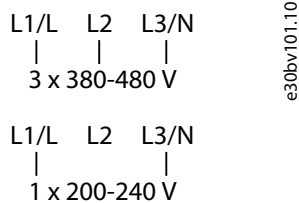
图解 39: 单相和三相接线
