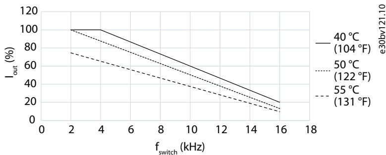
图解 17: 输出电流降额与开关频率的关系 (MA02a 3x380-480 V AC)
