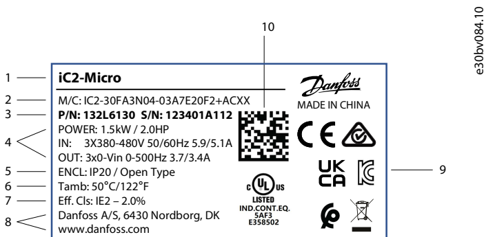
图解 21：产品标签示例
