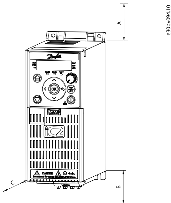
图解 27: 建议的维护通路间隙
