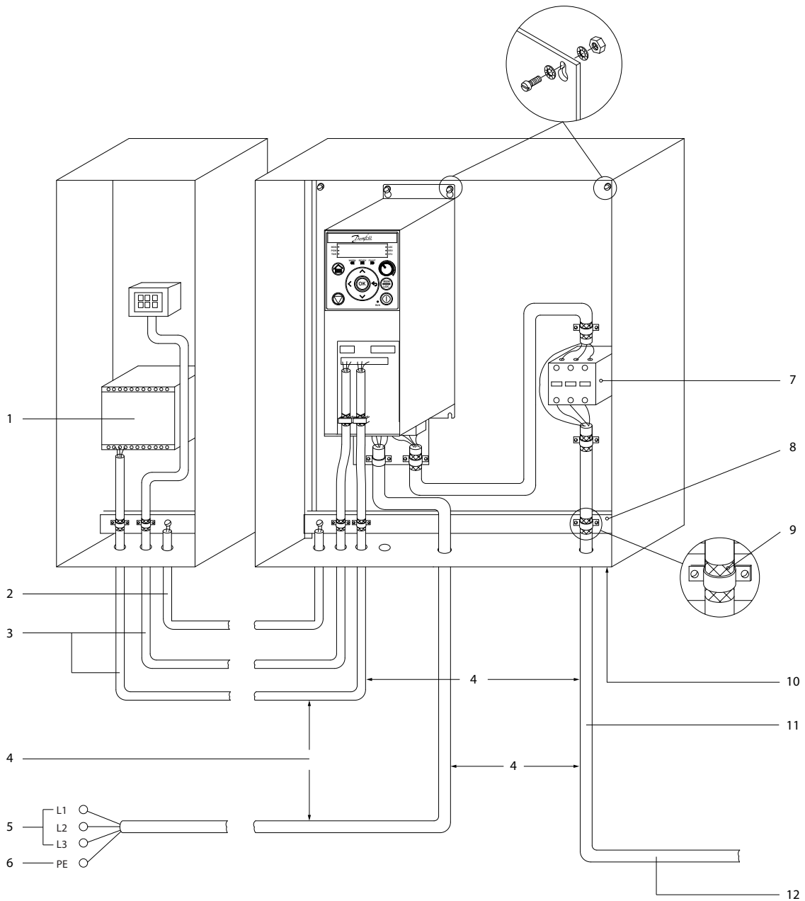
图解 30: 正确的 EMC 合规安装示例
