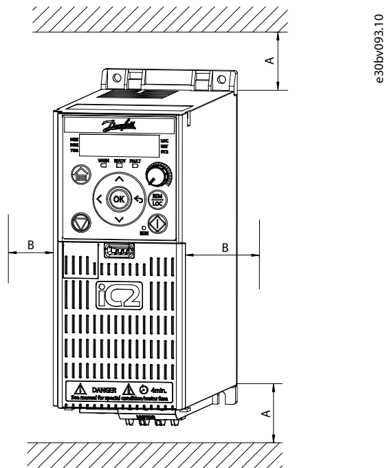
图解 26: 用于冷却的最小间隙
