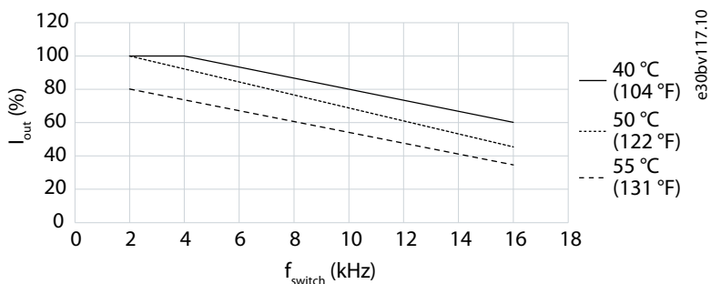
图解 13: 输出电流降额与开关频率的关系 (MA01c 1x200 - 240 V AC)
