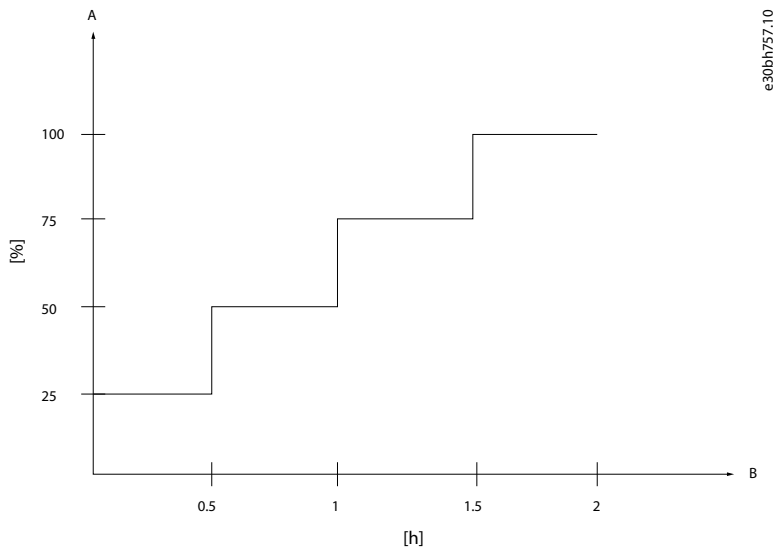
图解 23: 直流电容器的重整步骤
