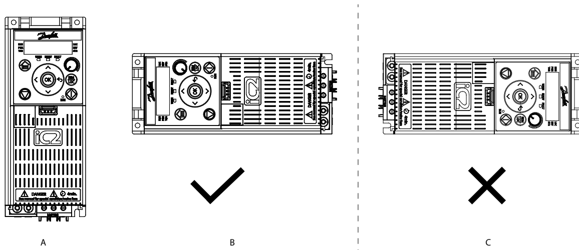
图解 24: 变频器的安装方向
