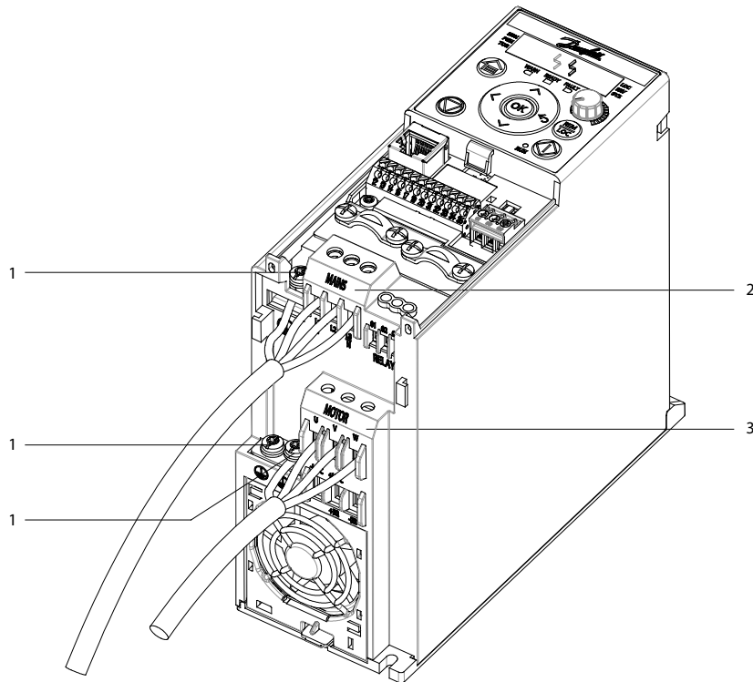
图解 38: 三相设备的主电源、电机和接地 (以 MA02a 为例)
